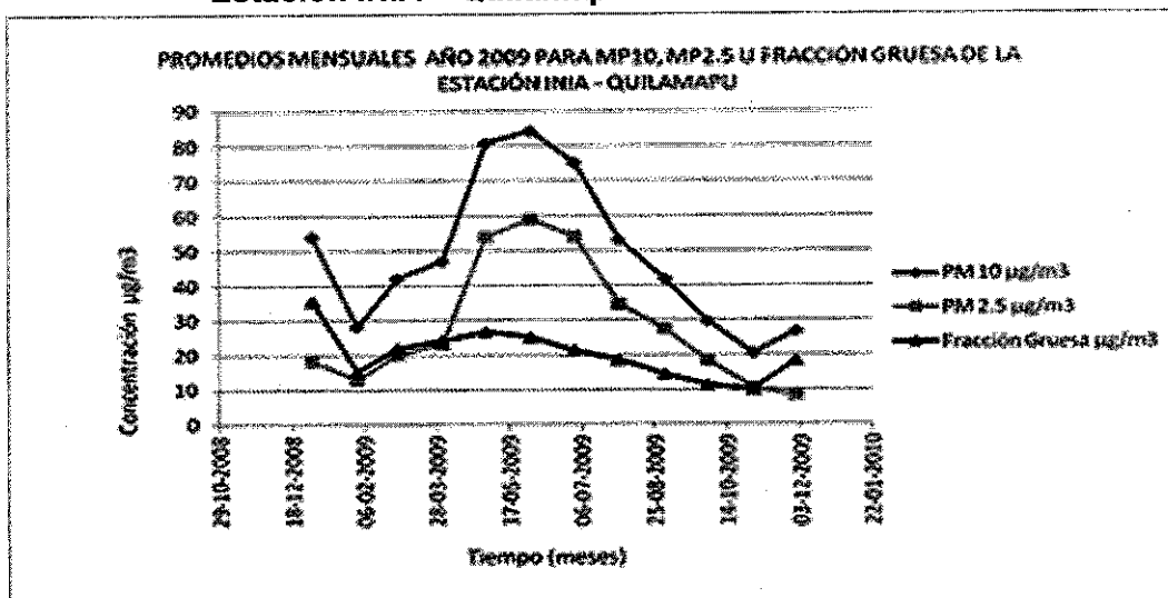
Figura N°6. Promedios mensuales del material particulado fino y grueso. Estación INIA – Quilamapu de Chillán – año 2009.
