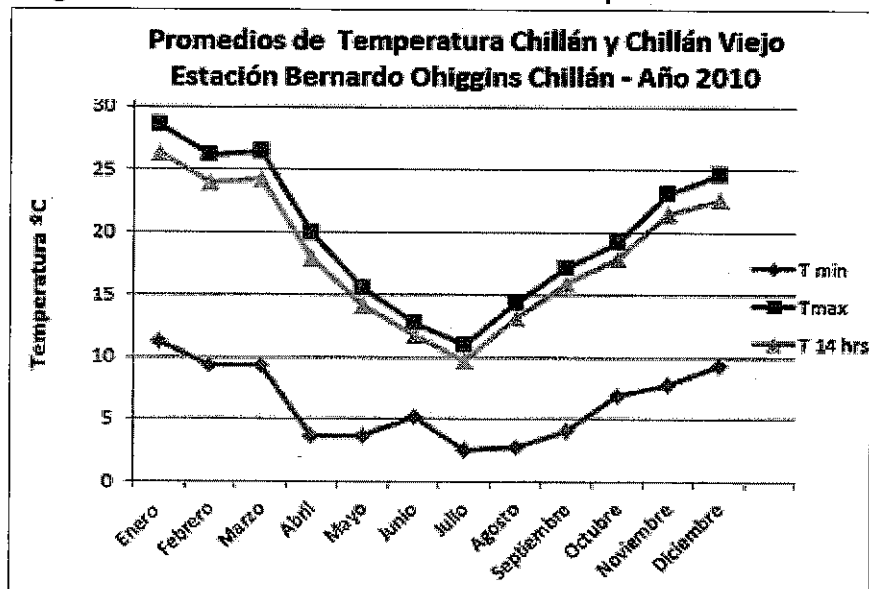
Figura N°1. Promedios mensuales de temperatura Año 2010
