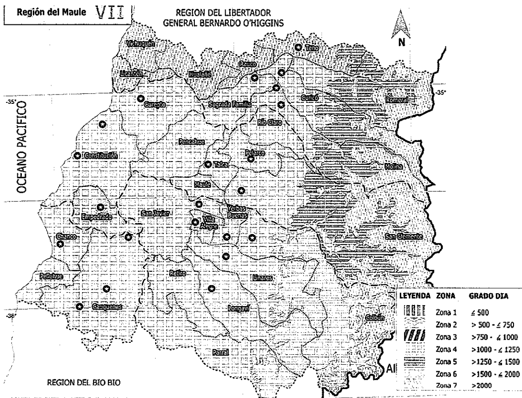
Figura 4: Zonas Térmicas de la Región del Maule.
